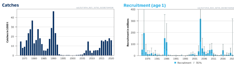
Figur 1. Fangster fra 1911-2020 udenskærs i Øst- og Sydgrønland (venstre). Indeks for 1-årige (højre).
